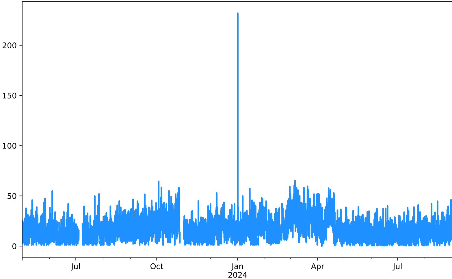
PM2.5 Estación MED-TESO Desde 2023-05-01 00:00 Hasta 2024-08-31 23:00
