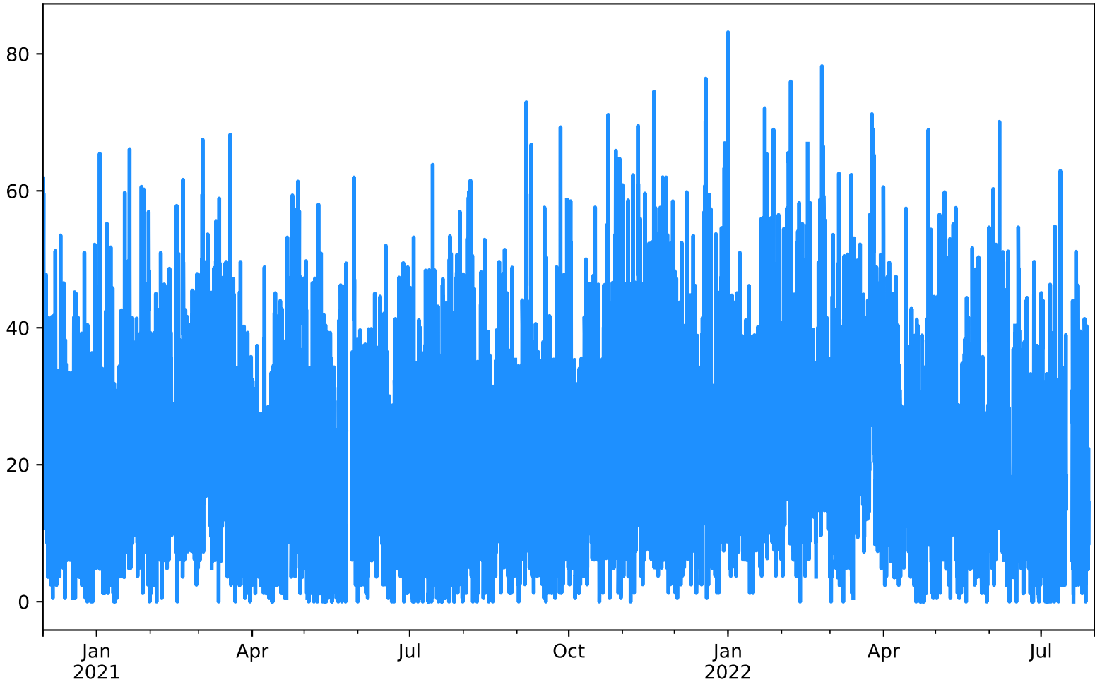
PM2.5 Estación MED-BEME Desde 2020-12-01 00:00 Hasta 2022-07-31 23:00
