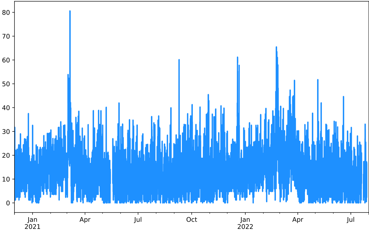
PM2.5 Estación COP-CVID Desde 2020-12-01 00:00 Hasta 2022-07-31 23:00
