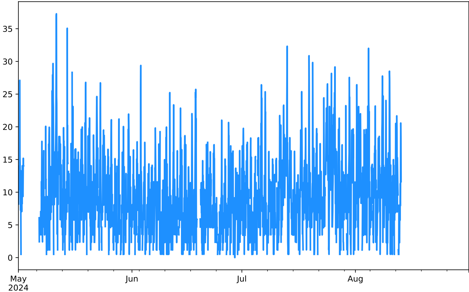
PM2.5 Estación BAR-TORR Desde 2024-05-01 00:00 Hasta 2024-08-31 23:00
