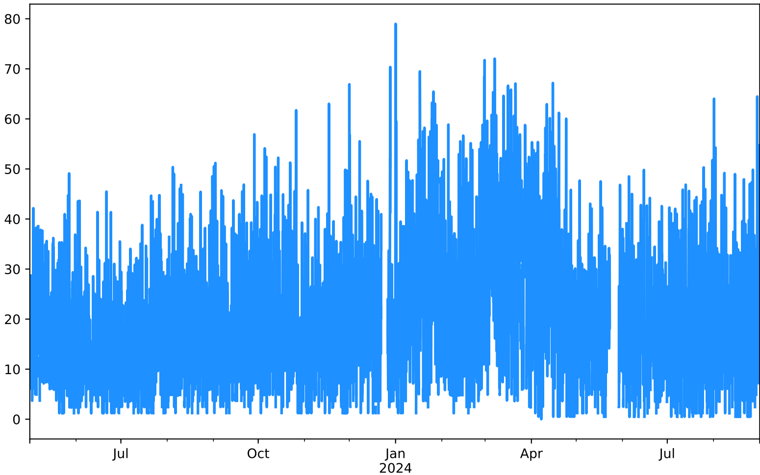
PM2.5 Estación MED-ALTA Desde 2023-05-01 00:00 Hasta 2024-08-31 23:00
