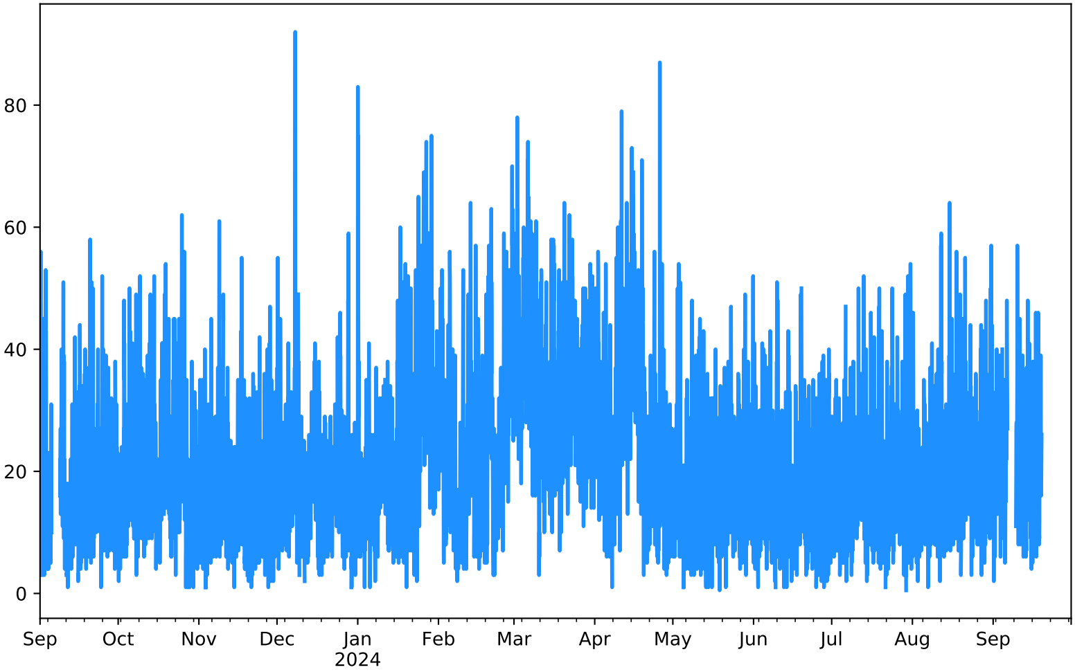
PM2.5 Estación ITA-CJUS Desde 2023-09-01 00:00 Hasta 2024-09-30 23:00
