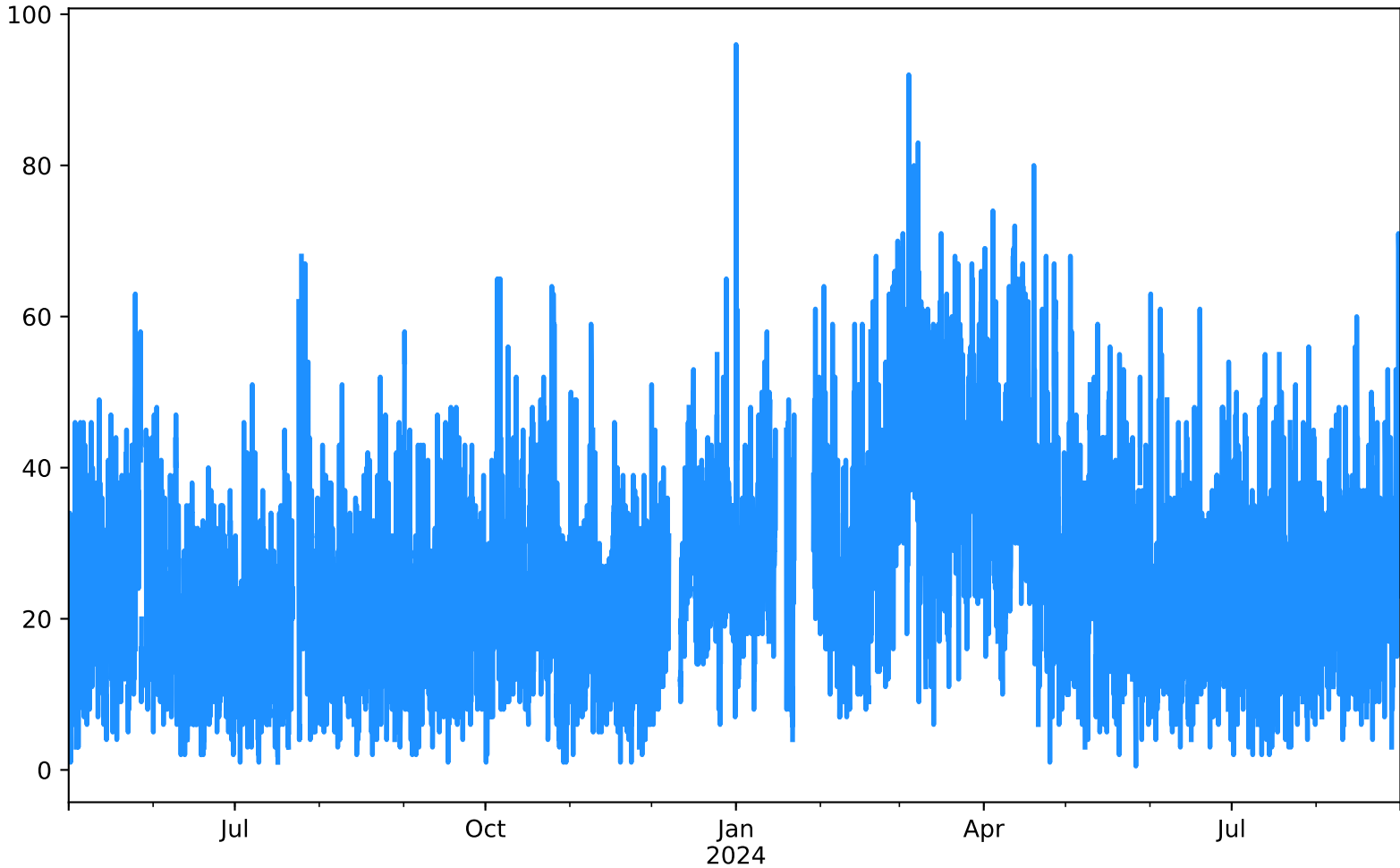
PM2.5 Estación CEN-TRAF Desde 2023-05-01 00:00 Hasta 2024-08-31 23:00
