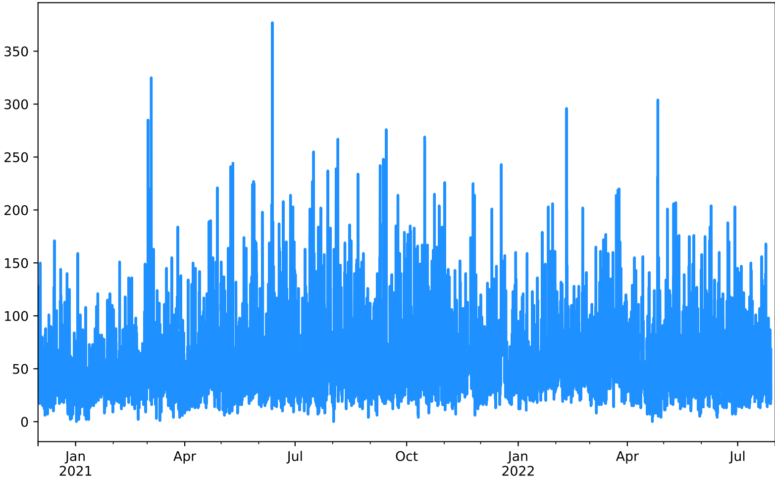
PM10 Estación ITA-POGO Desde 2020-12-01 00:00 Hasta 2022-07-31 23:00
