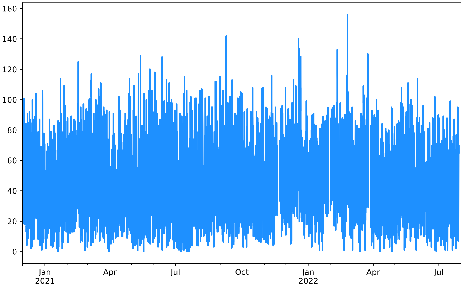
PM10 Estación MED-EXSA Desde 2020-12-01 00:00 Hasta 2022-07-31 23:00
