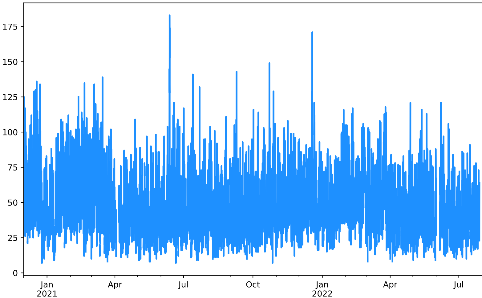
PM10 Estación CEN-TRAF Desde 2020-12-01 00:00 Hasta 2022-07-31 23:00
