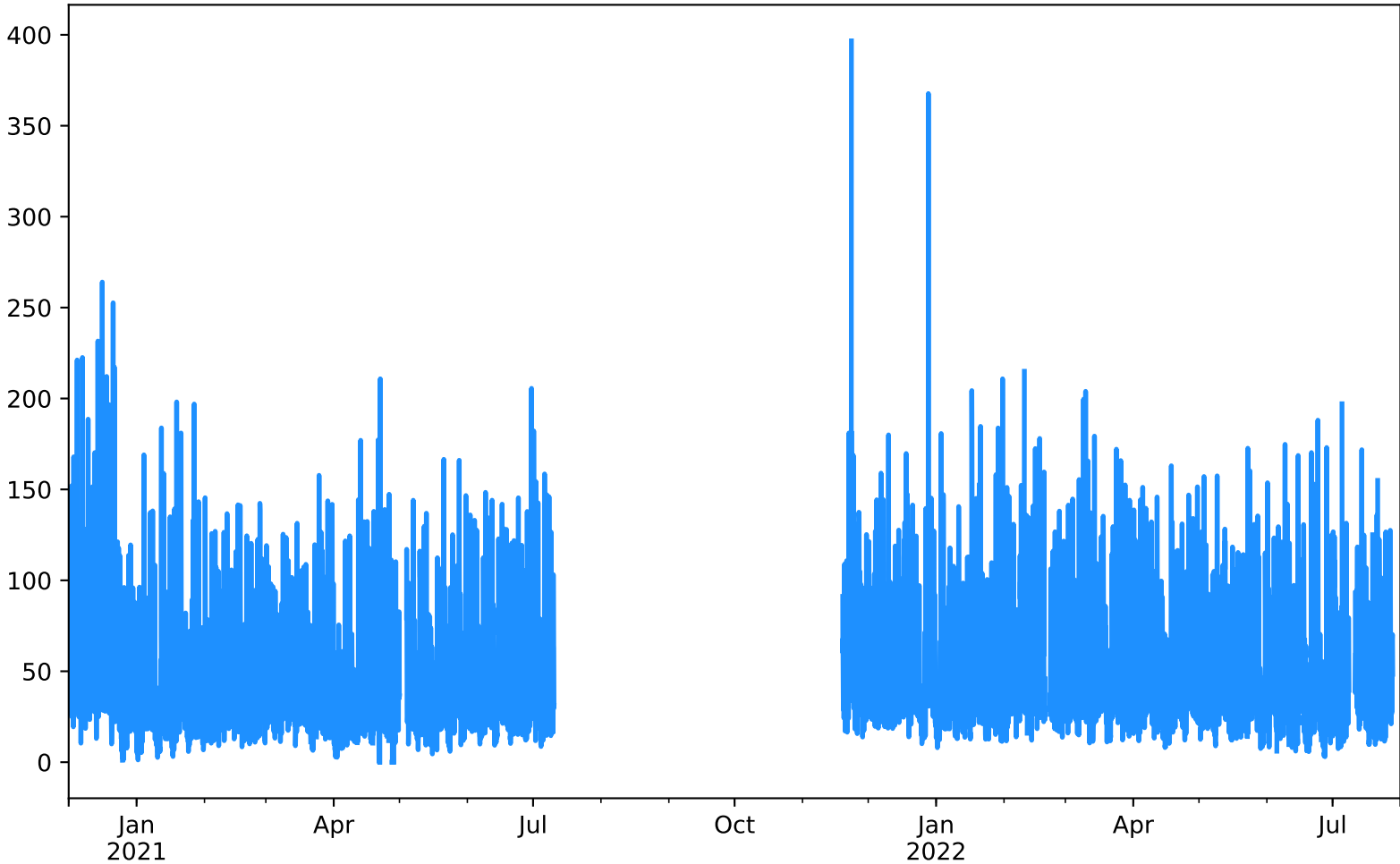
NOx Estación SUR-TRAF Desde 2020-12-01 00:00 Hasta 2022-07-31 23:00
