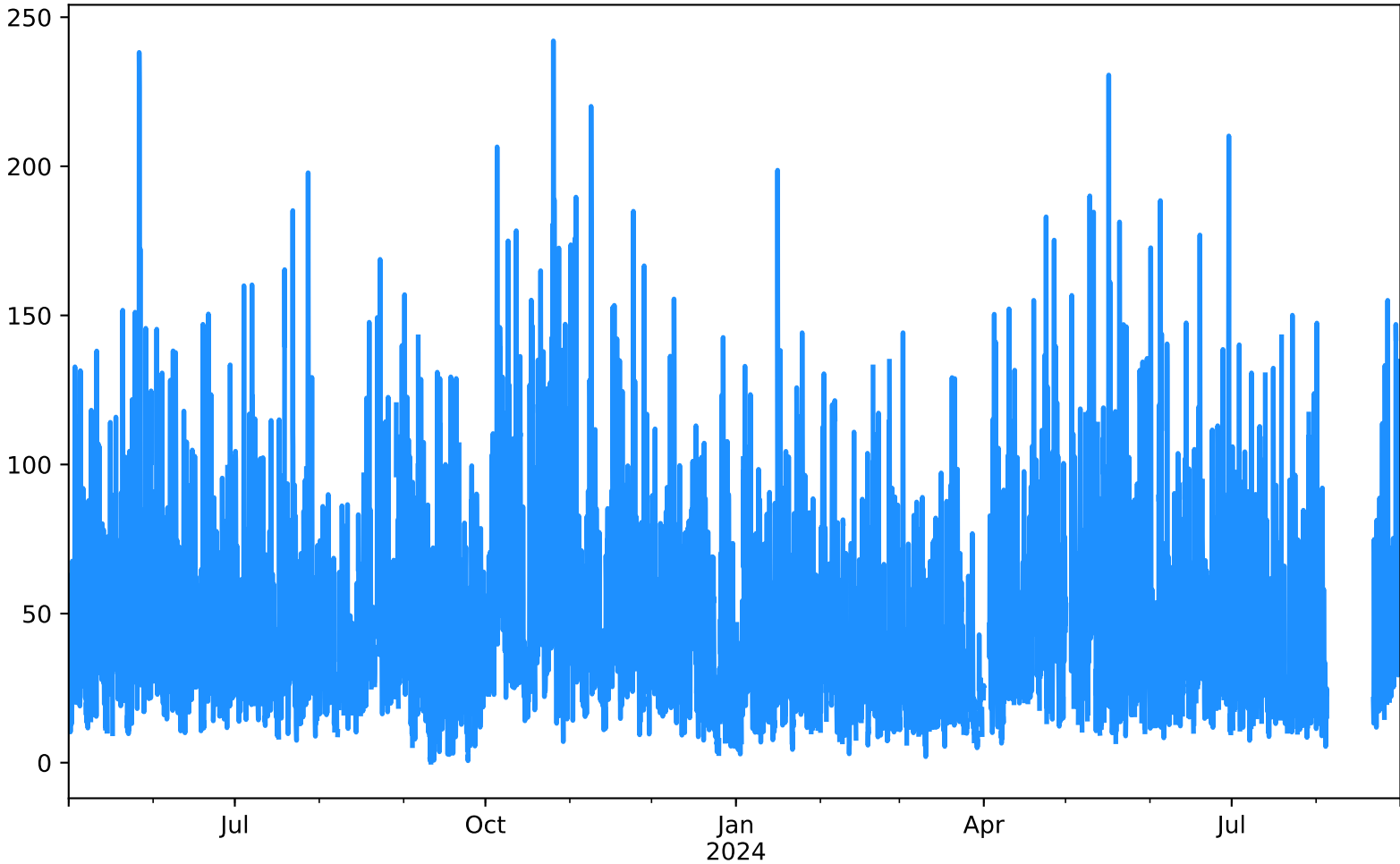
NOx Estación CEN-TRAF Desde 2023-05-01 00:00 Hasta 2024-08-31 23:00
