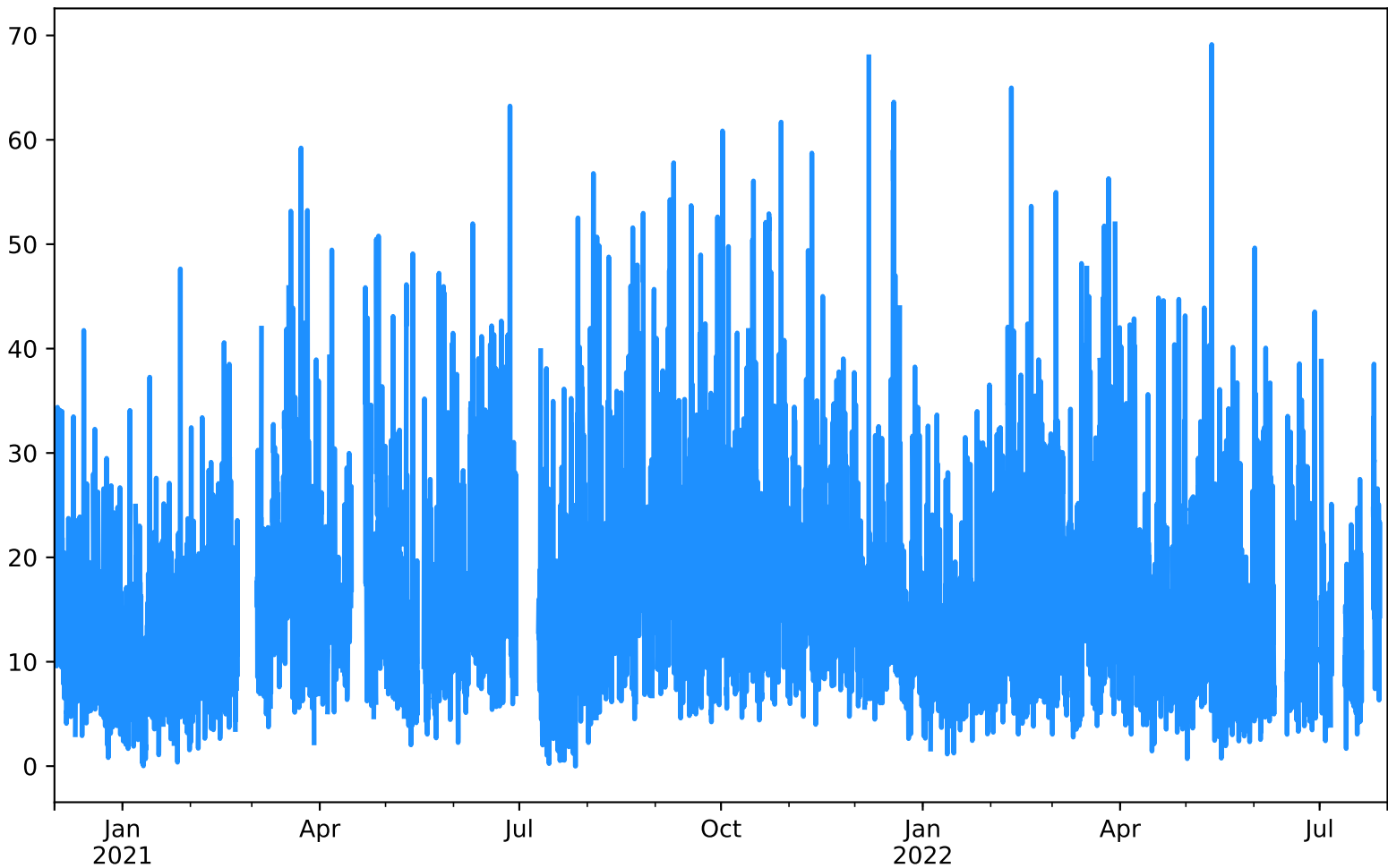
NO2 Estación MED-ITMR Desde 2020-12-01 00:00 Hasta 2022-07-31 23:00
