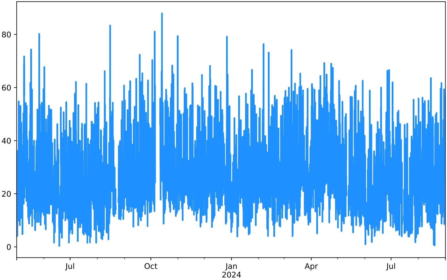
NO2 Estación MED-PJIC Desde 2023-05-01 00:00 Hasta 2024-08-31 23:00
