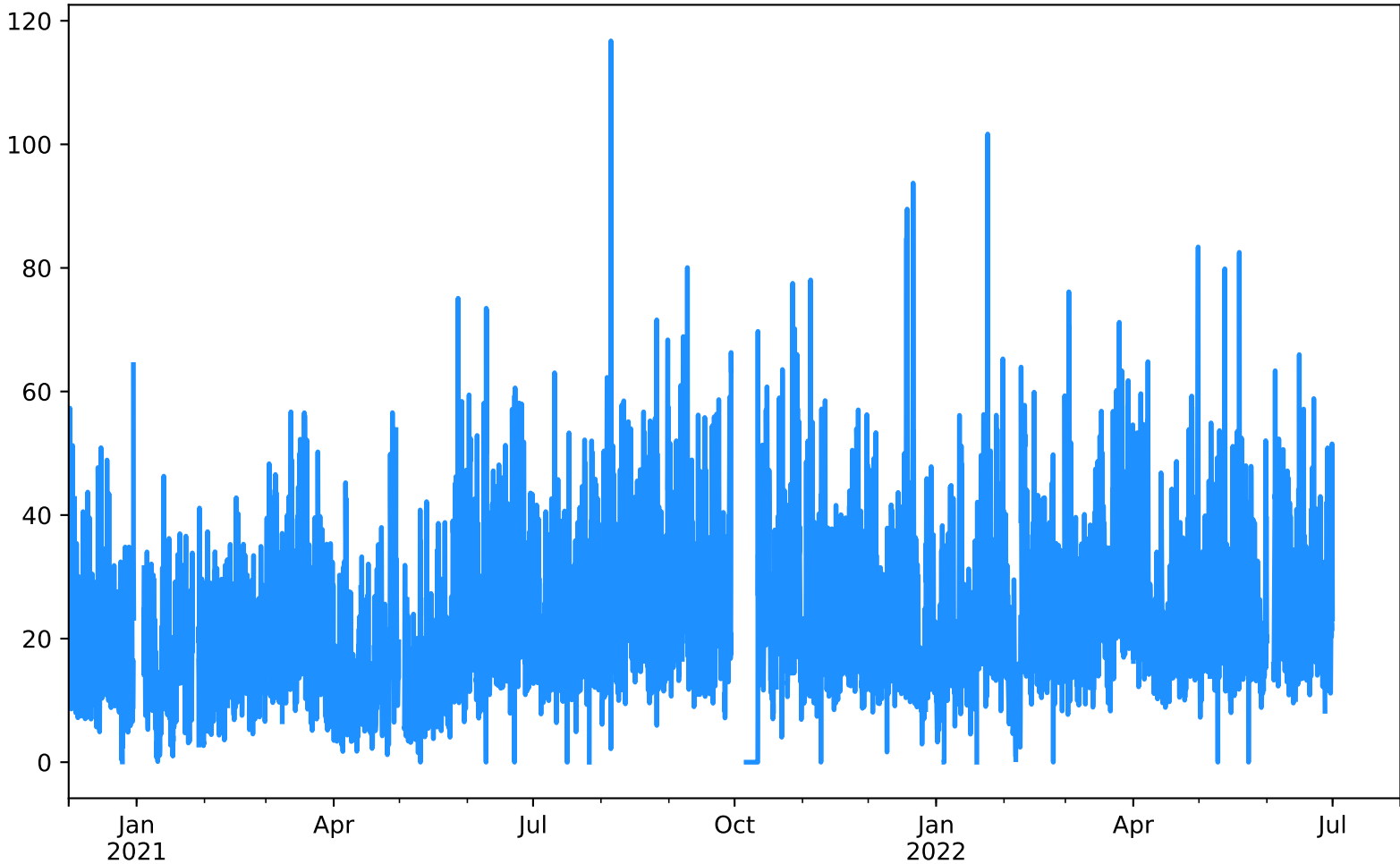
NO2 Estación CEN-TRAF Desde 2020-12-01 00:00 Hasta 2022-07-31 23:00
