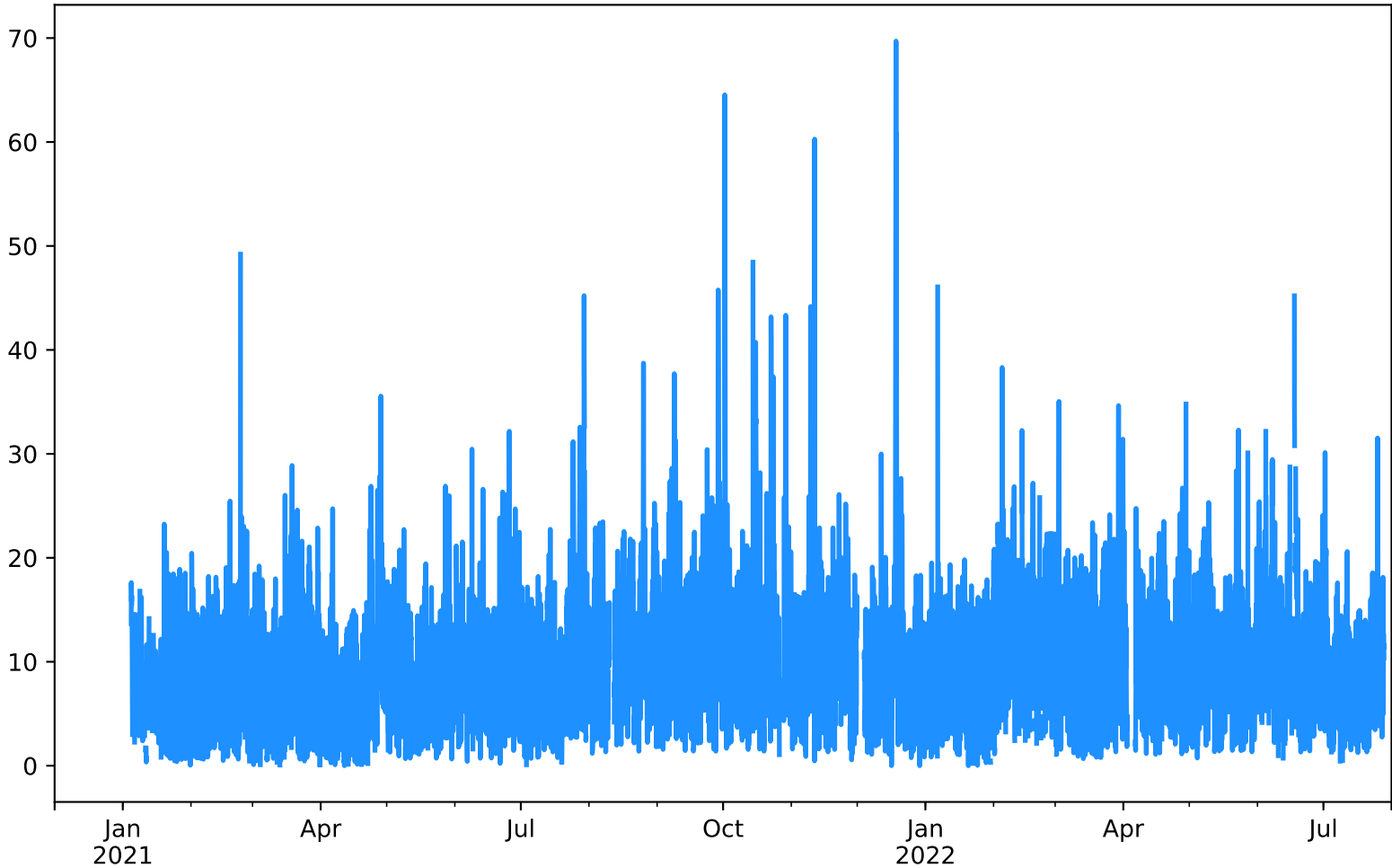
NO2 Estación GIR-EPM Desde 2020-12-01 00:00 Hasta 2022-07-31 23:00
