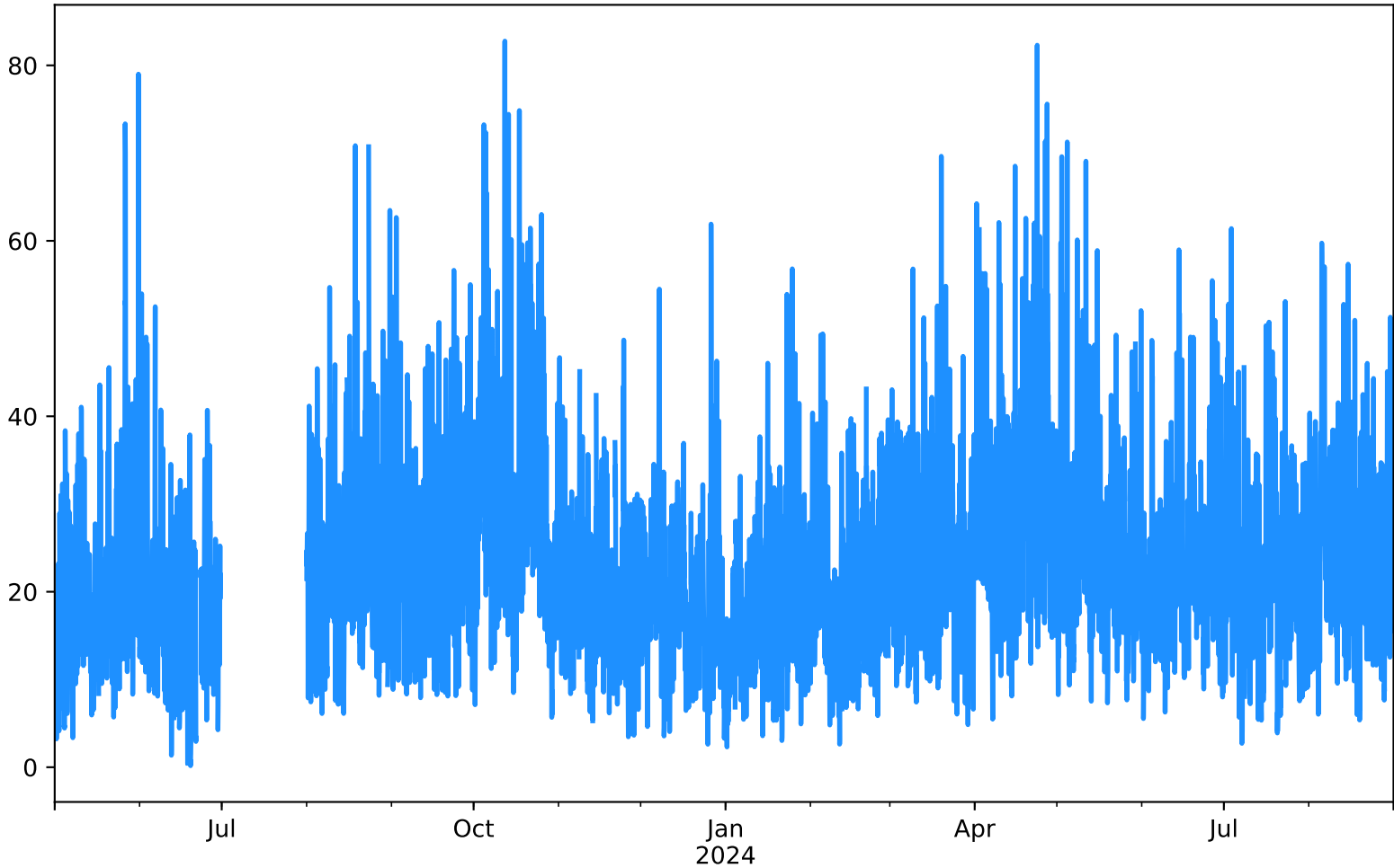
NO2 Estación MED-FISC Desde 2023-05-01 00:00 Hasta 2024-08-31 23:00
