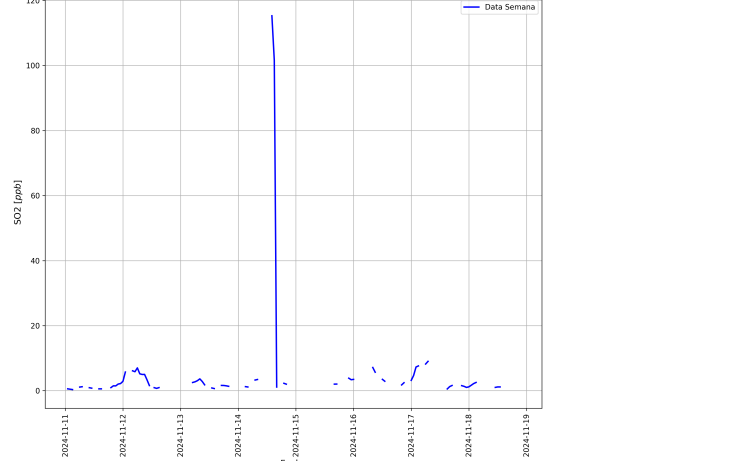
SO2 Estación MED-FISC Desde 2024-11-11 01:00 Hasta 2024-11-19 00:00
