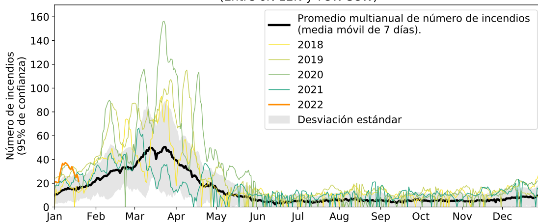
Datos de Incendios/Hotspots MODIS (Collection 6) 2001 - 2022 Noreste de Colombia y Venezuela (Entre 6N 12N y 78W 58W)
