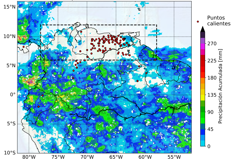
Datos de Puntos Calientes/Hotspots MODIS (Collection 6) 2001 - 2025 Noreste de Colombia y Venezuela (Entre 6N 12N y 78W 58W)
