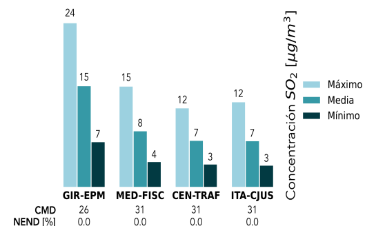
Figura 19. Estadísticos del mes a partir de promedios diarios asociados a SO 2 .
