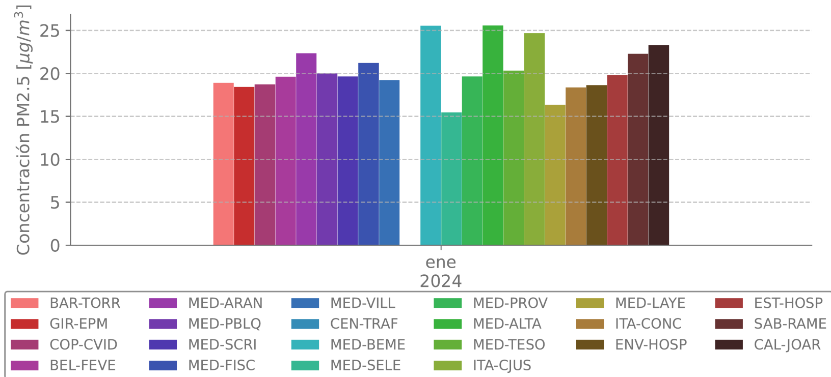
Figura 5. Concentraciones mensuales asociados a PM2.5.
