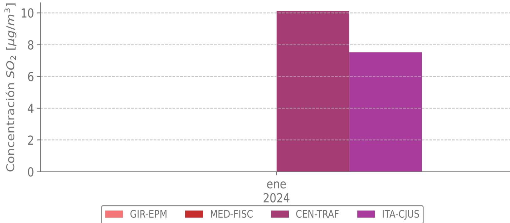
Figura 21. Concentraciones mensuales asociados a SO_2 .
