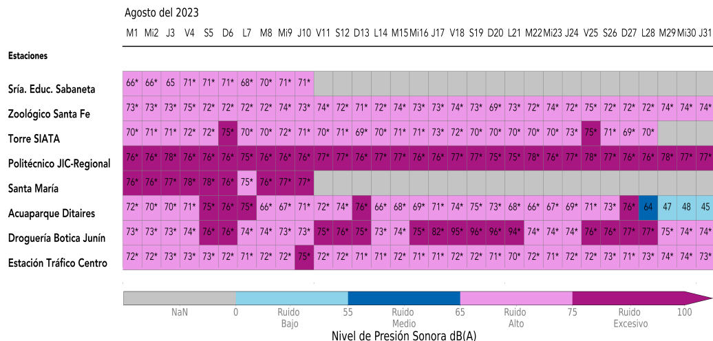
Figura 22. Nivel de Presión Sonora Día Noche para las estaciones de monitoreo de Ruido Ambiental.
