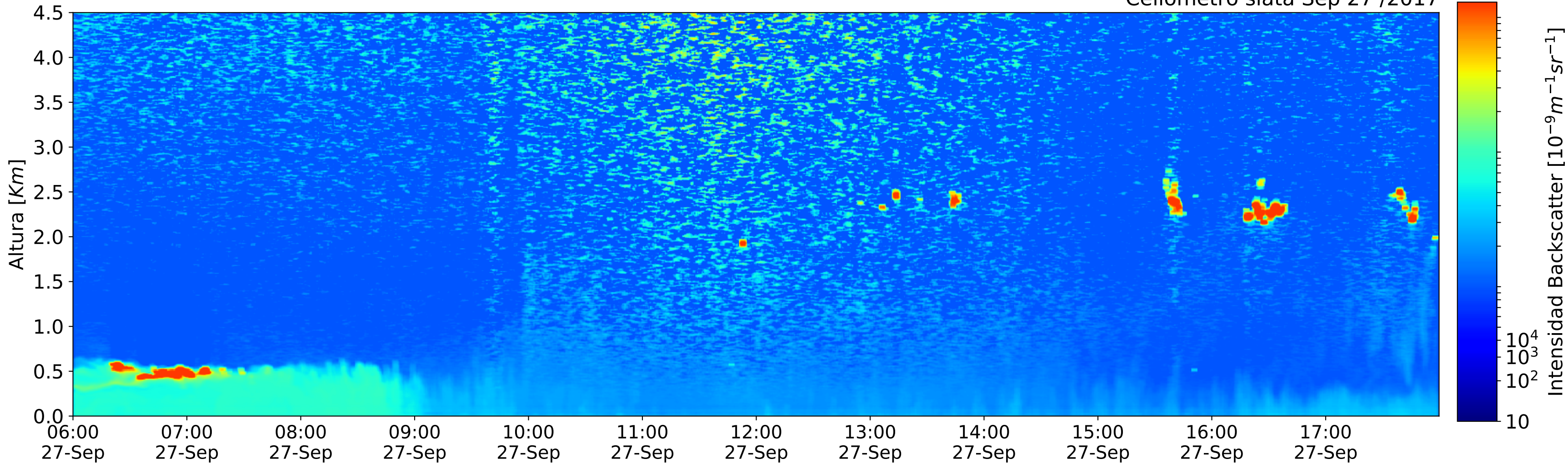
Ceilometro siata Sep 27 /2017
