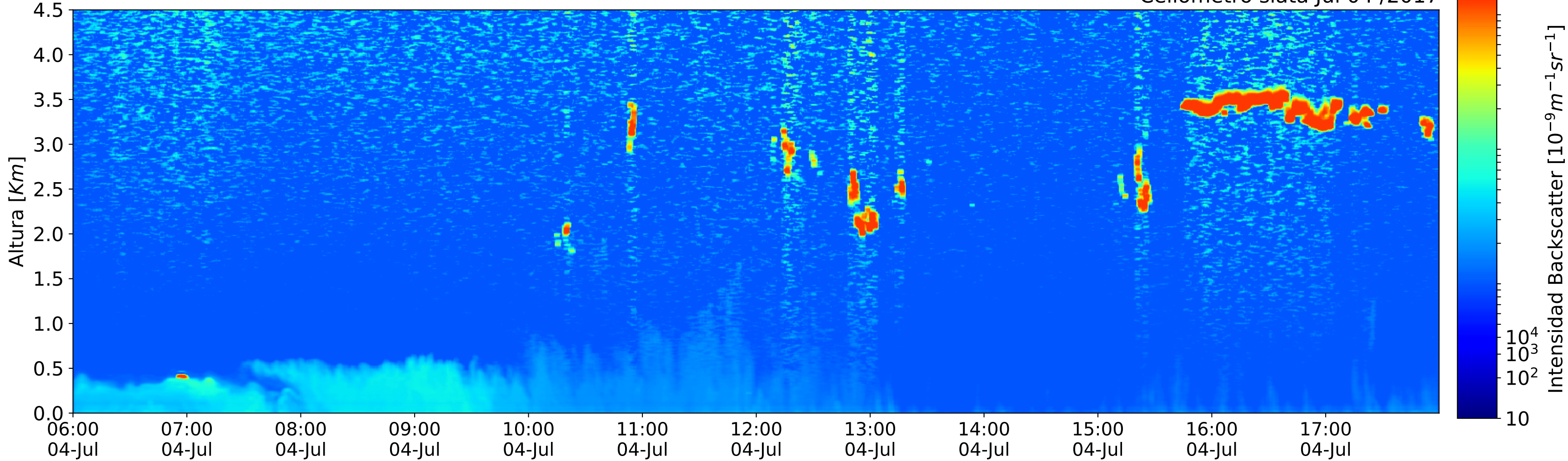
Ceilometro siata Jul 04 /2017
