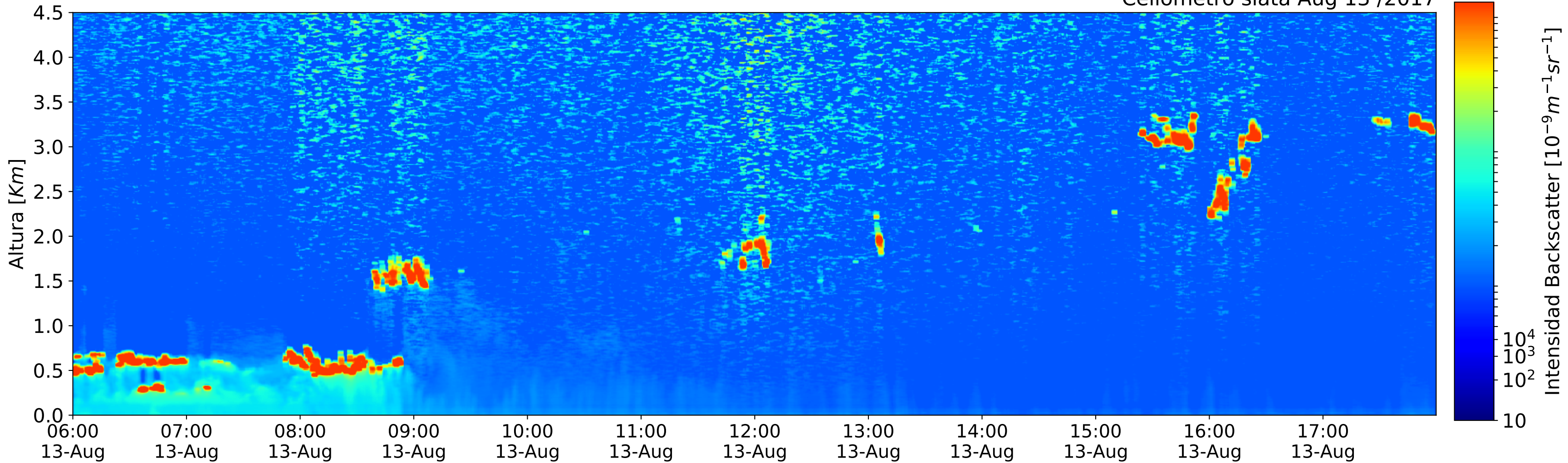
Ceilometro siata Aug 13 /2017
