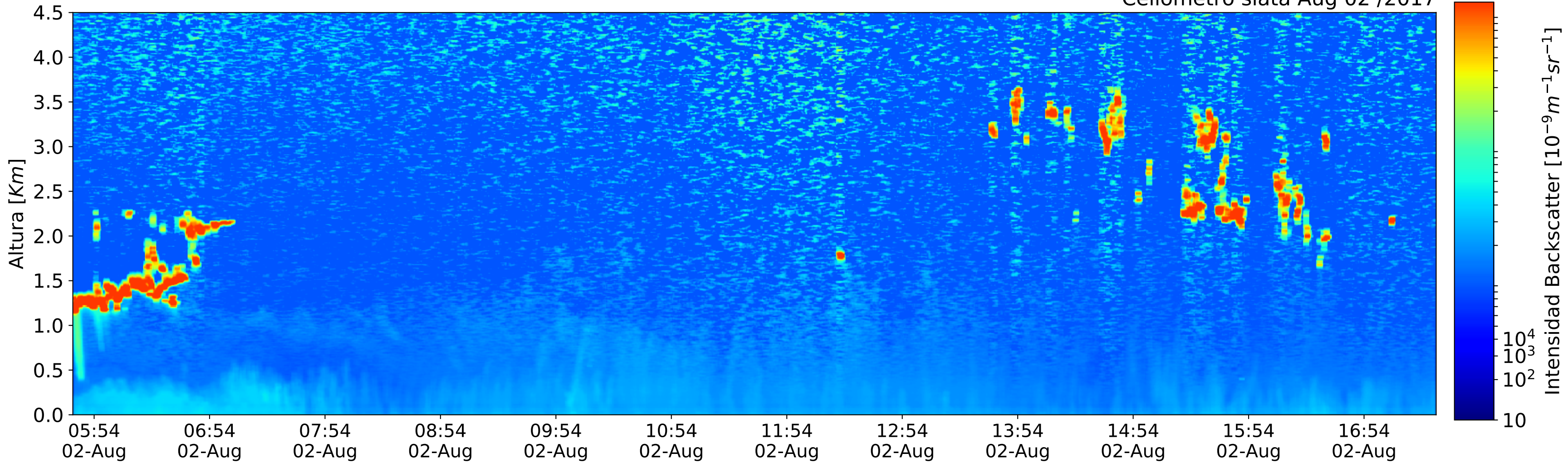
Ceilometro siata Aug 02 /2017
