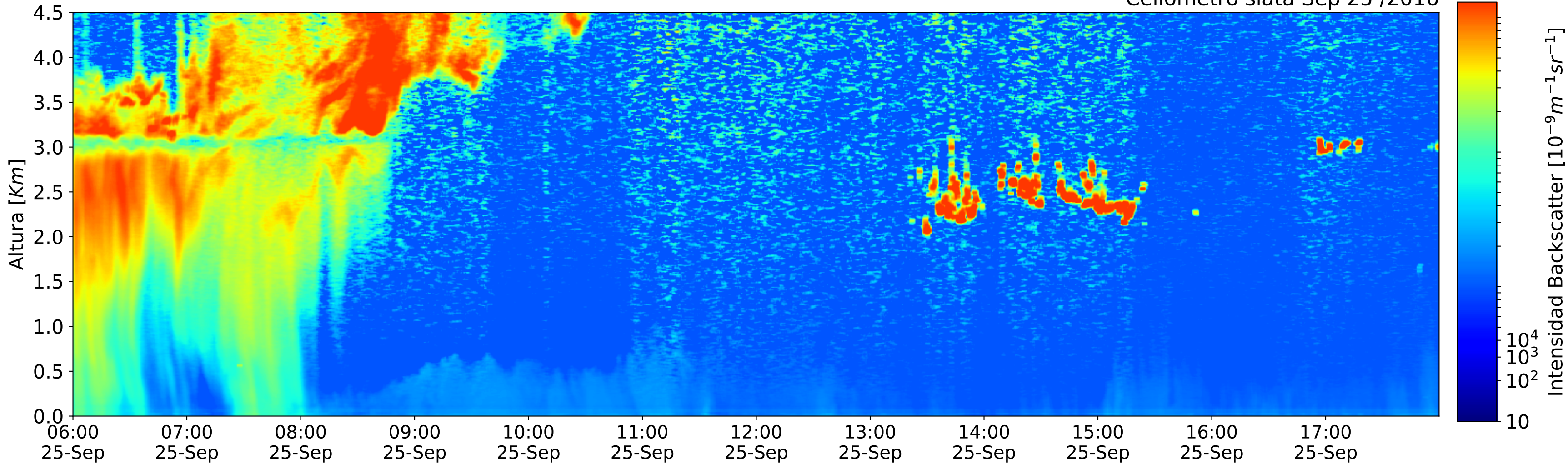
Ceilometro siata Sep 25 /2016
