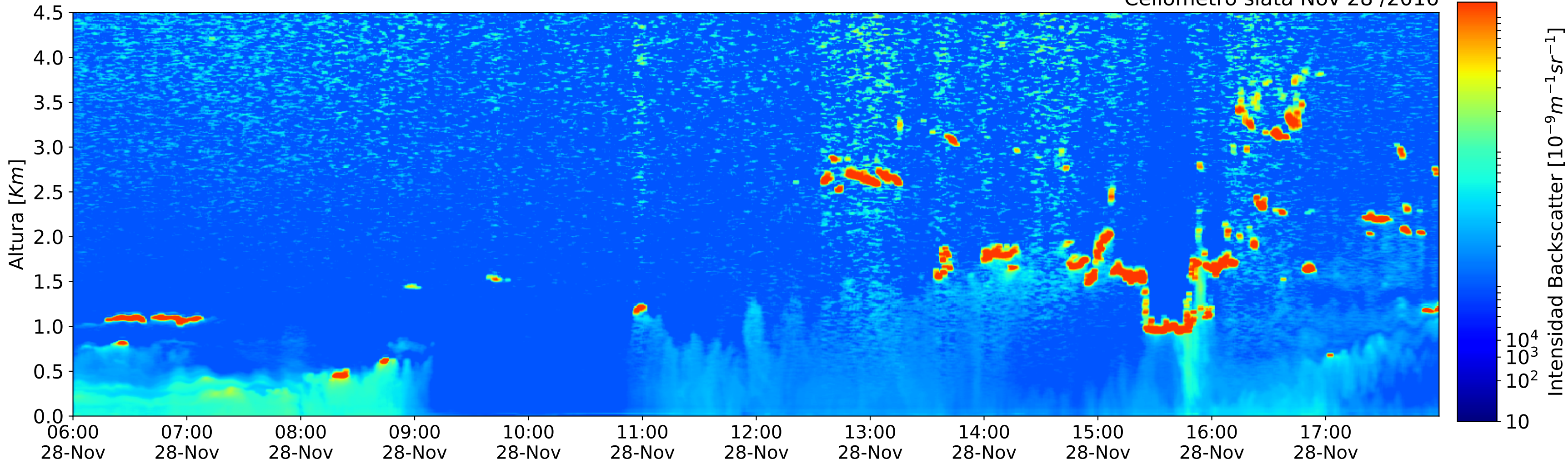
Ceilometro siata Nov 28 /2016
