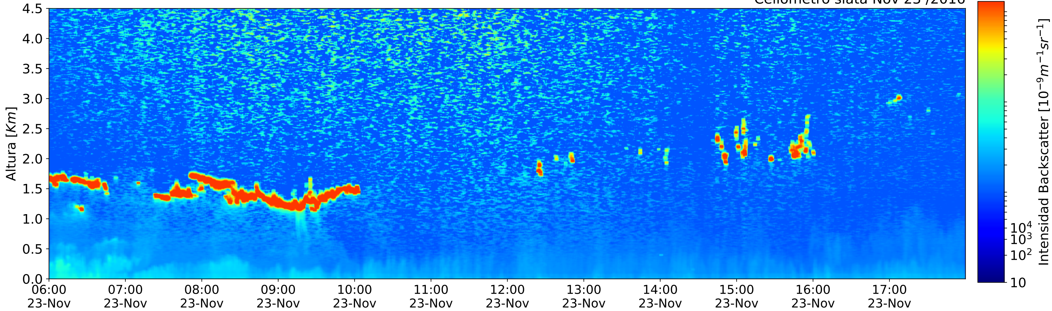
Ceilometro siata Nov 23 /2016
