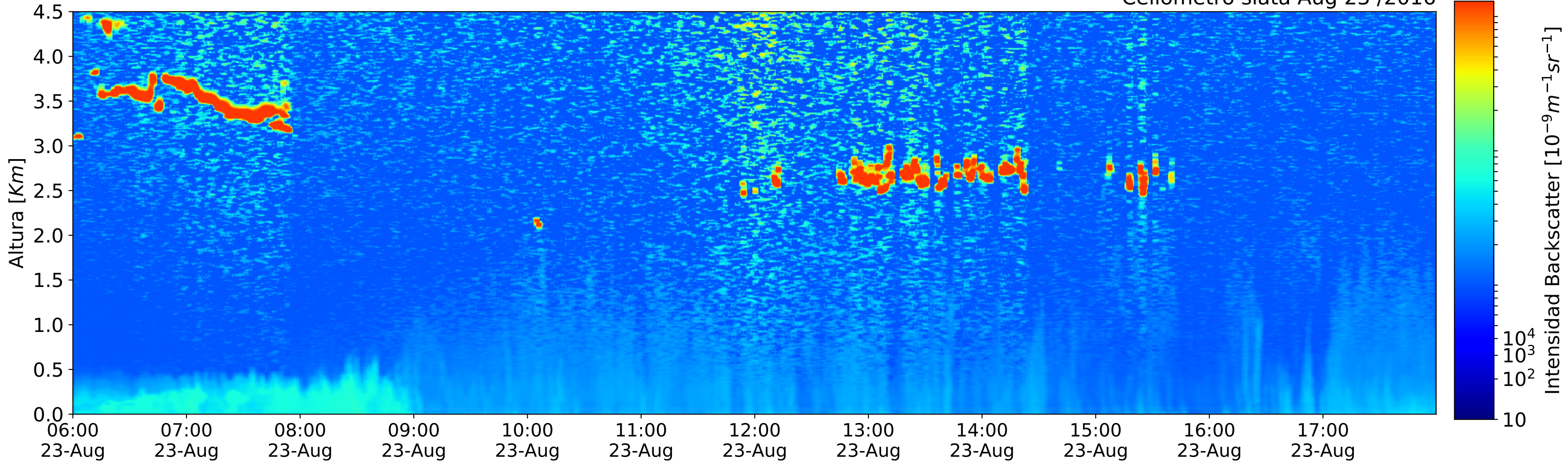
Ceilometro siata Aug 23 /2016
