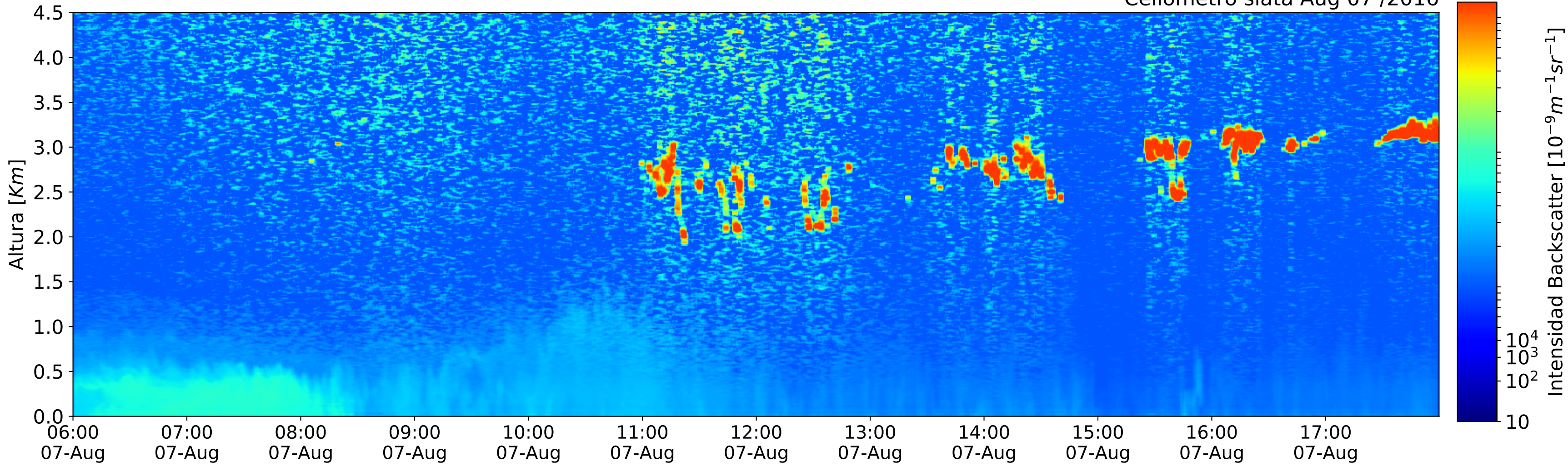
Ceilometro siata Aug 07 /2016
