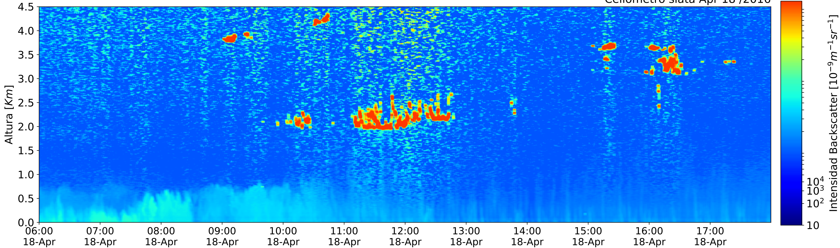
Ceilometro siata Apr 18 /2016
